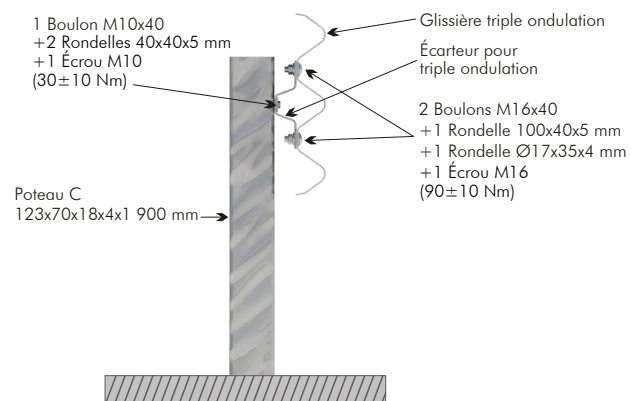
Détail de la liaison du poteau intermédiaire
